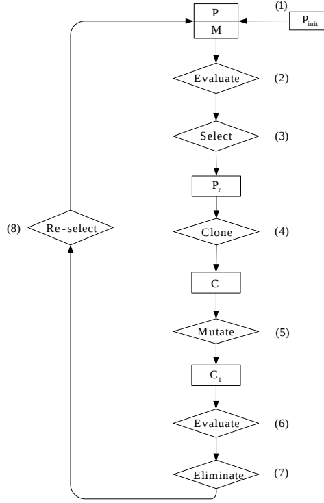
Fig. 1. Flow chart of basic CSA.
